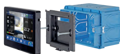
Instalación empotrada 503
