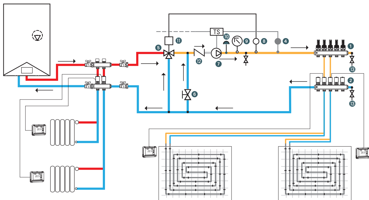
TM3-R termostático con colectores con medidores de caudal (4 l/min), baja temperatura
